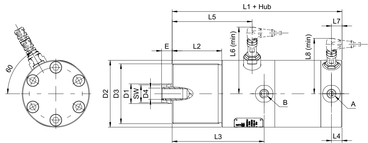
Maße und Kräfte Baureihe CYPULL CP-HR-P / CP-HR-L
